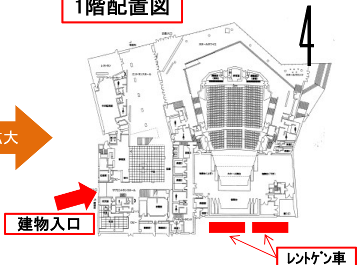
1階配置図
